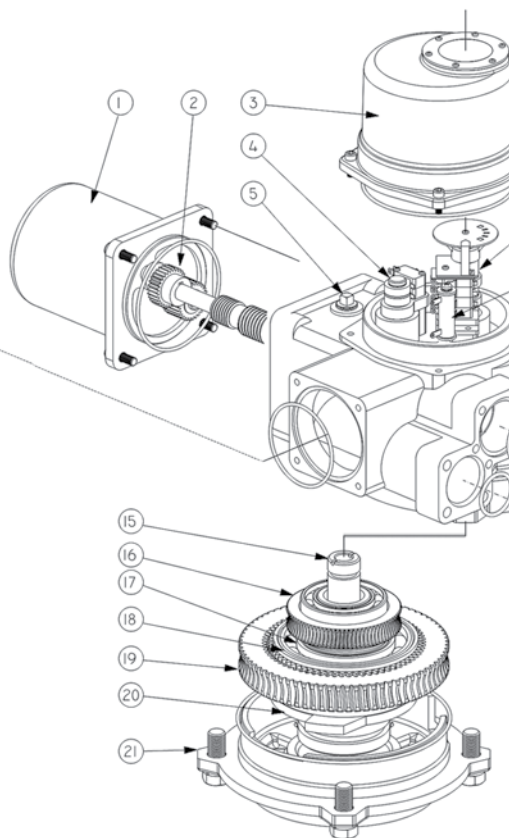
Рис.1 Электропривод ГЗ-ОФ
